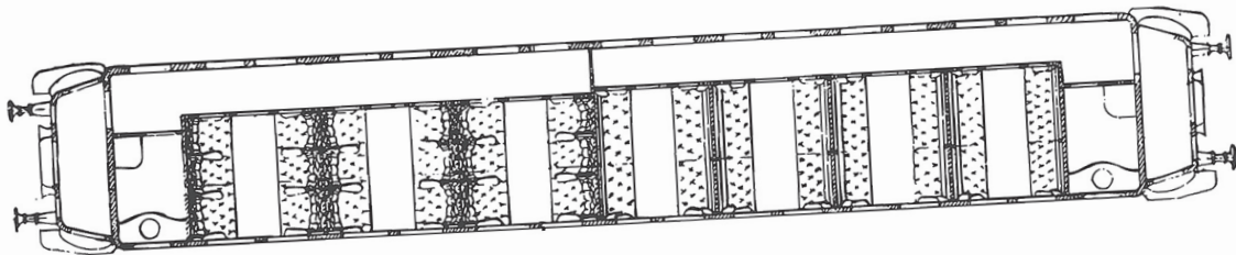
Plan d'une voiture de première et seconde classe à couloir.
